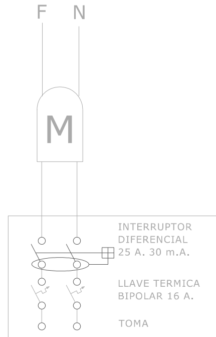
DIAGRAMA DE CONEXION
